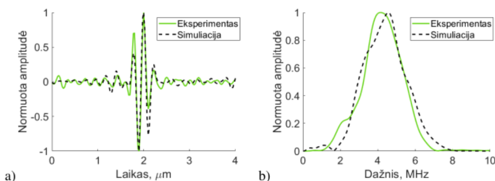
3.1 pav. Eksperimento ir simuliacijos palyginimas: a) aido impulso signalai atsispindėję nuo 15 mm gylyje esančios vielutės (ašinis vaizdas), b) aido impulso signalų spektrai
