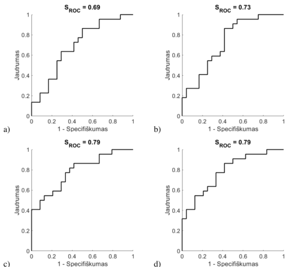
3.9 pav. ROC kreivės a) spektrinio centro, b) spektrinės sklaidos, c) spektrinės asimetrijos, d) spektrinio eksceso parametrų vertinant jų diagnostinę vertę nustatant aterosklerozę
