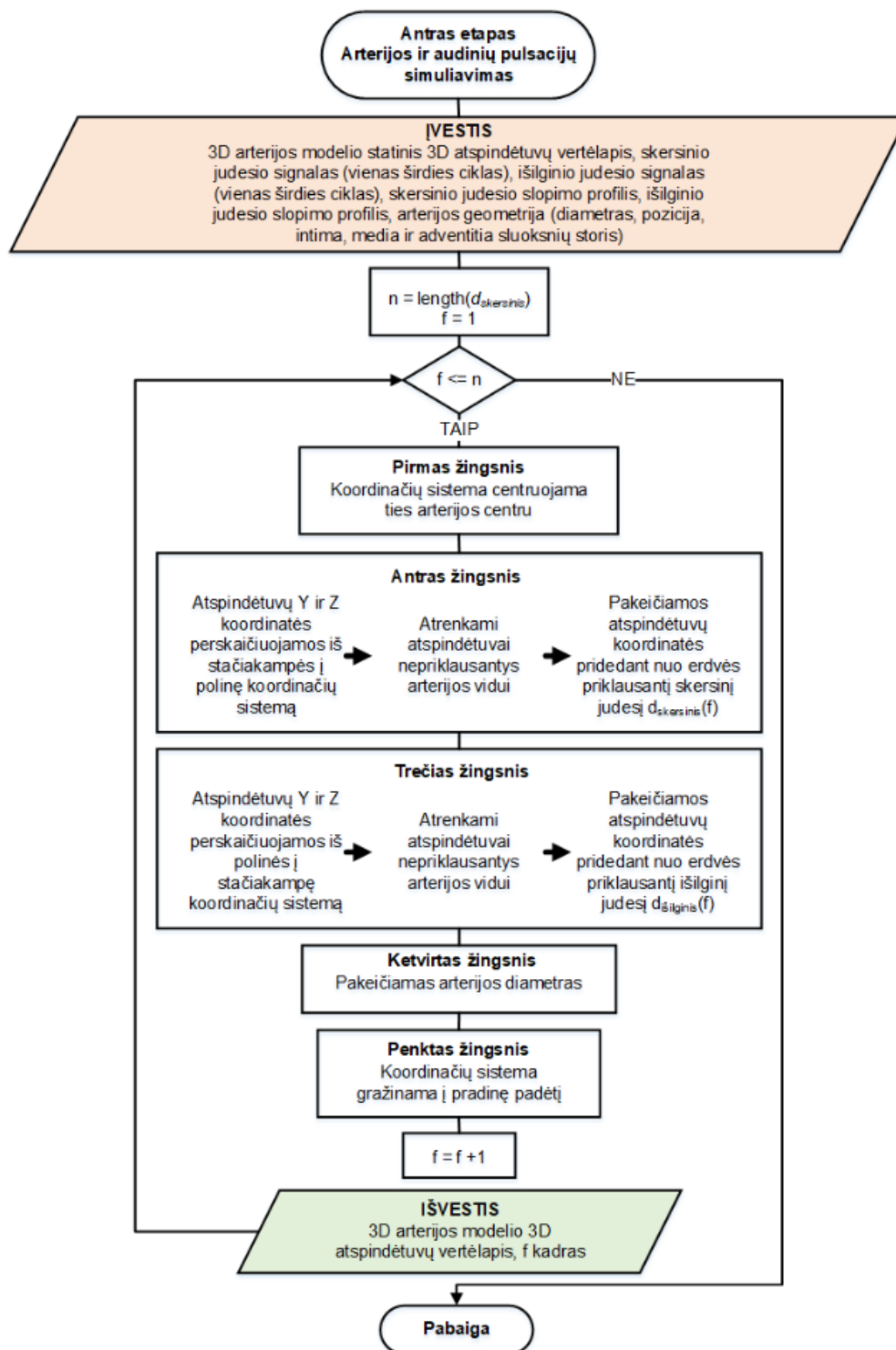
2.7 pav. Funkcinė antro etapo schema, simuliuoti kompleksinę arterijos ir audinių pulsaciją. Čia f atitinka šiuo metu analizuojamą kadro skaičių judesio signalė ir n - bendrą tokių kadro skaičių
