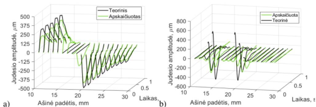
3.5 pav. Viršutinės ir apatinės arterijos sienelių ir aplinkinių audinių judesiai detektuoti su OpenOpticalFlow algoritmu, 23 metų moteris: a) 1 mm amplitudės teorinis ir apskaičiuotas skersinis judesys, b) 1 mm amplitudės teorinis ir apskaičiuotas išilginis judesys
