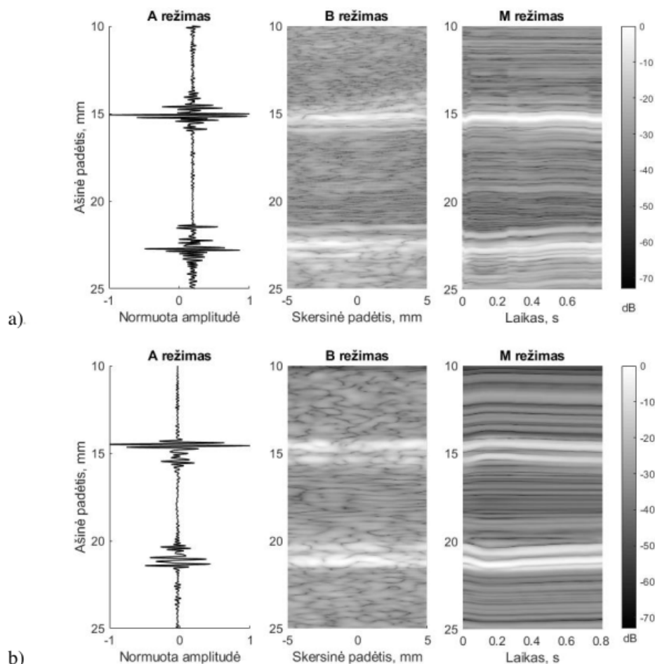
3.4 pav. Radiodažnių signalų formos palyginimas (A režimas, f_1 kadras, skersinė padėtis 0 mm), B režimo vaizdas ( f_1 kadras), judesys laike (M režimas): a) in vivo atvejis (23 metų moteris, judesio amplitudė nenormuota), b) simuliuotas atvejis (23 metų moteris, judesio amplitudė normuota į 1 mm)
