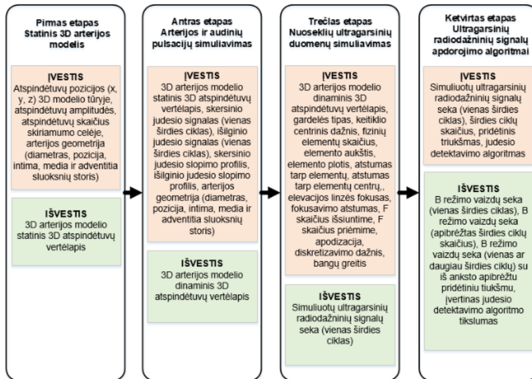
2.4 pav. Apibendrinta simuliacijos algoritmo eiga
