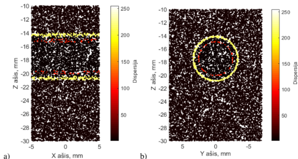
2.6 pav. 3D atspindėtuvų vertėlapis atvaizduojantis arterijos modelį iš skirtingų projekcijų: a) išilginė, b) ašinė
